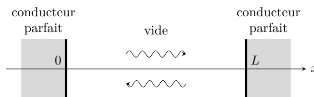
Figure 4 – Cavité électromagnétique formée par deux plans conducteurs.
