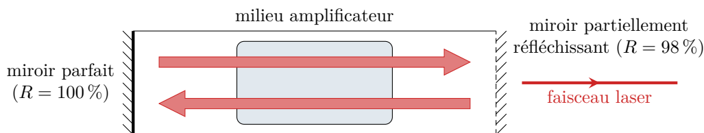
Figure 3 – Schéma de principe d'un laser. Dans un laser, une onde électromagnétique est confinée dans une cavité formée de deux miroirs contenant un milieu amplificateur. À chaque passage dans le milieu amplificateur, l'onde est amplifiée. L'un des miroirs est imparfait, ce qui permet à l'onde électromagnétique de sortir du laser.
