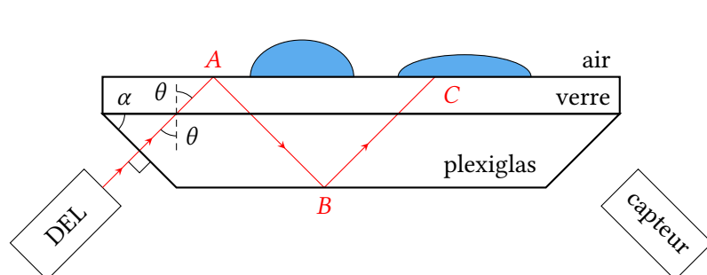
Figure 1 – Principe de fonctionnement d'un détecteur de pluie.
