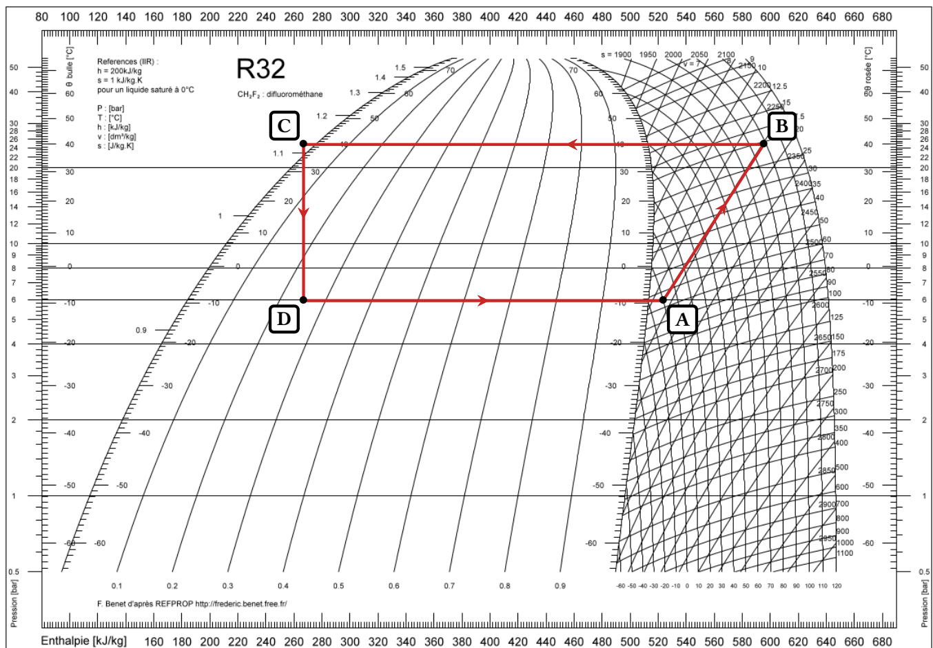
Figure 7 – Cycle de la PAC représenté dans le diagramme des frigoristes du R32. On remarque que le cycle est parcouru en sens trigonométrique, ce qui est caractéristique d'une machine réceptrice dans tous les diagrammes et pas seulement dans le diagramme de Watt.
