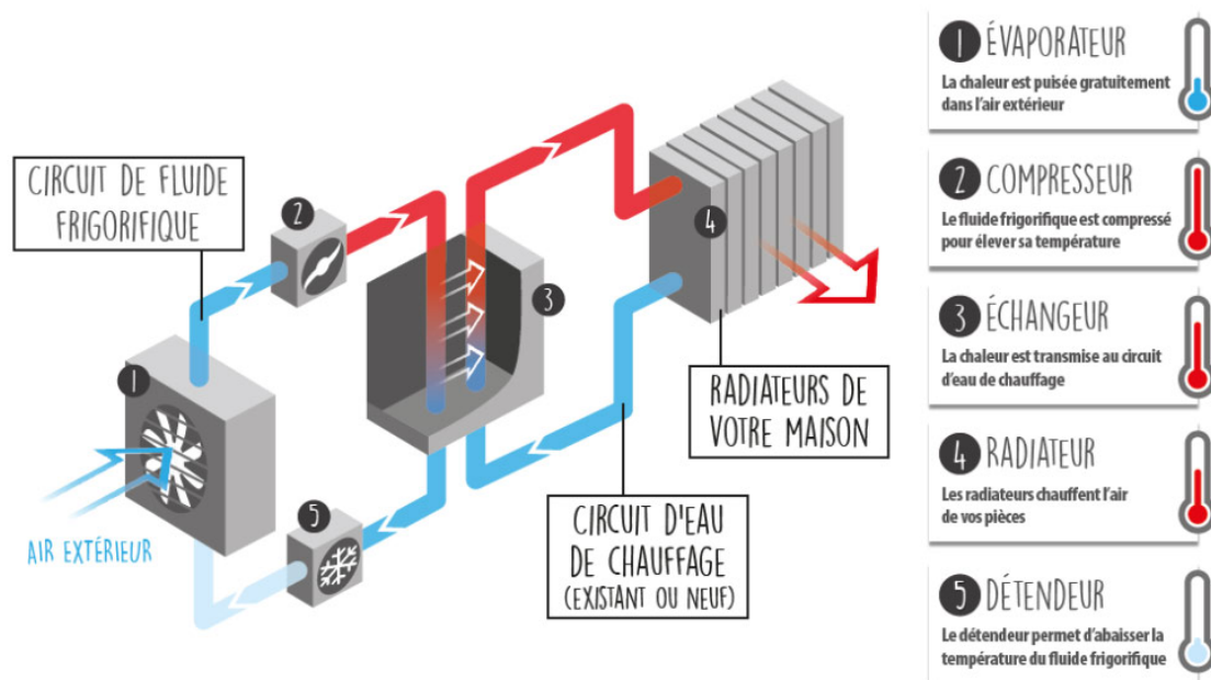
Figure 6 – Schéma explicatif du principe d'une PAC air-eau. Dans une PAC air-eau, la source froide est l'air extérieur, et la source chaude l'eau du circuit de chauffage. Dans le principe, un climatiseur fonctionne à l'identique, en inversant « l'intérieur » et « l'extérieur » de la maison. Schéma issu d'un site de fabricant.
