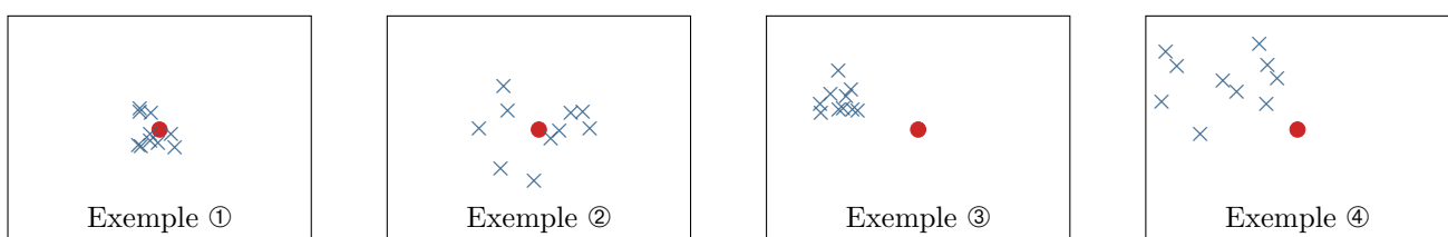
Figure 2 – Représentation schématique de quatre protocoles expérimentaux.
