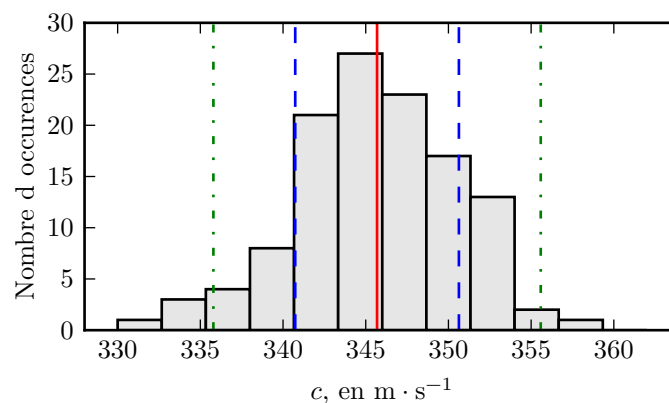
Figure 3 – Histogramme des résultats expérimentaux issus de 120 mesures. La hauteur de chaque rectangle indique le nombre de résultats dont la valeur est comprise entre les deux extrémités de la base. Le trait continu rouge indique la valeur moyenne, les traits pointillés sont séparés d'un écart-type.
