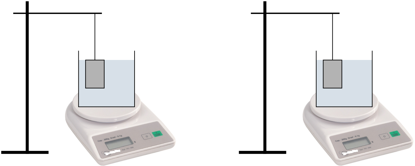
Figure 1 – Dispositif expérimental de mesure de la poussée d'Archimède.
