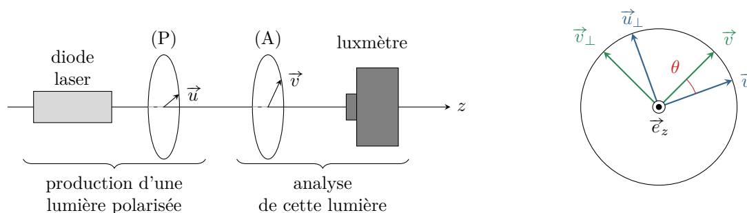
Figure 1 – Production et analyse d'une polarisation rectiligne.
